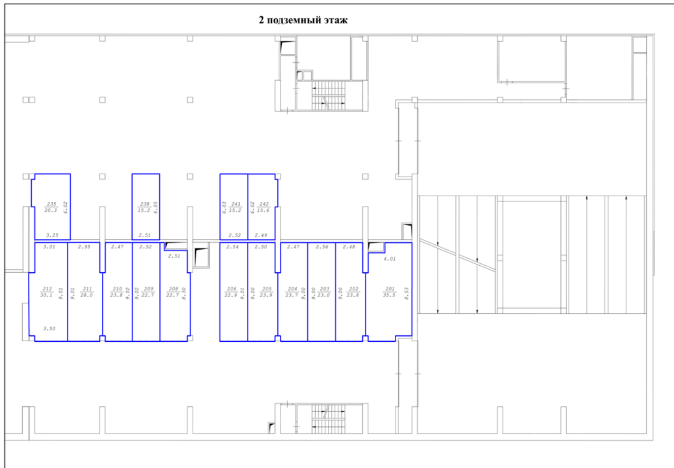
Фрагмент графической части проекта технического плана образуемых машино-мест
