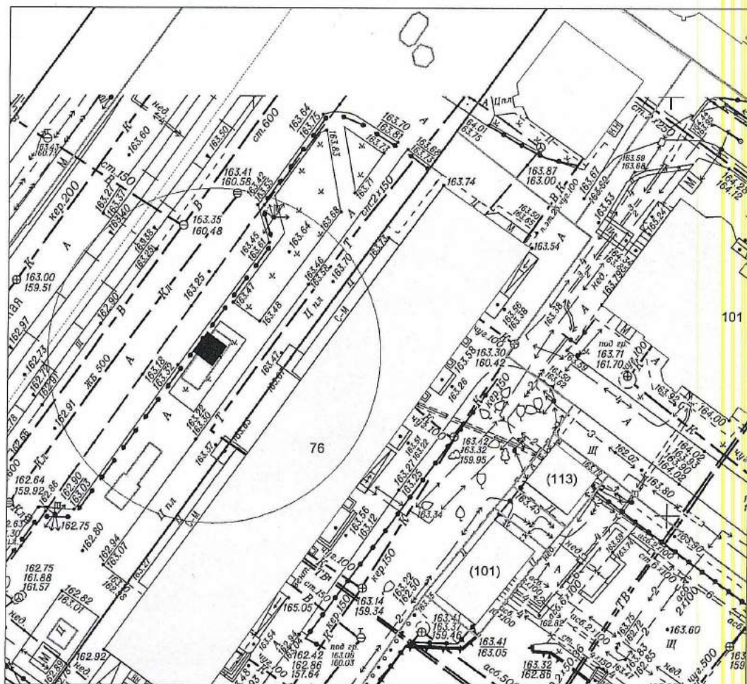
Схема к акту № 817 по адресному ориентиру ул. Гурьевская, (76) на топографическом плане М1:500
