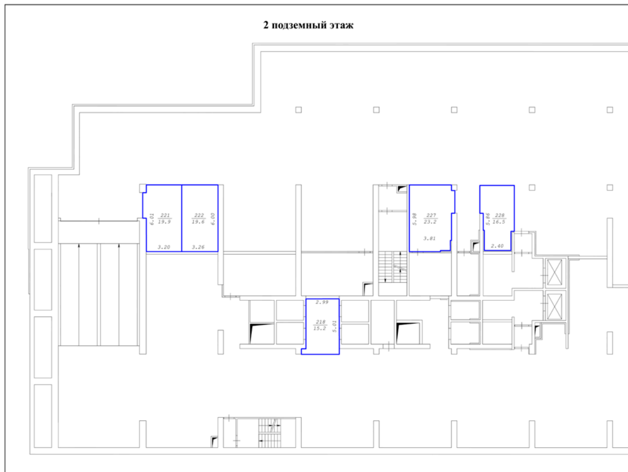
Фрагмент графической части проекта технического плана образуемых машино-мест
